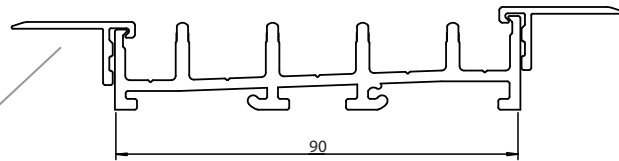
UNTERE FÜHRUNGSSCHIENE, 4-SPURIG
