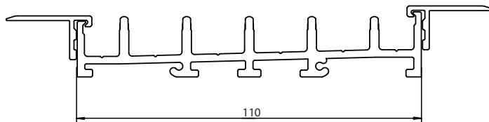
UNTERE FÜHRUNGSSCHIENE, 5-SPURIG
