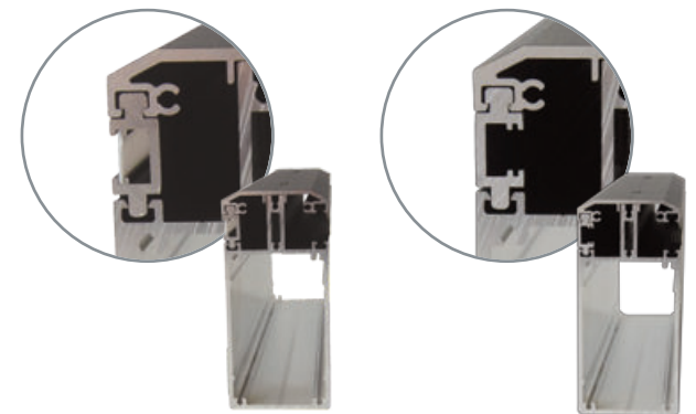
Multifunktionales Abschlussprofil der Außensparren: entweder als Abschlußprofil einsetzbar oder für den integrierten Einsatz von LED Stripes.
